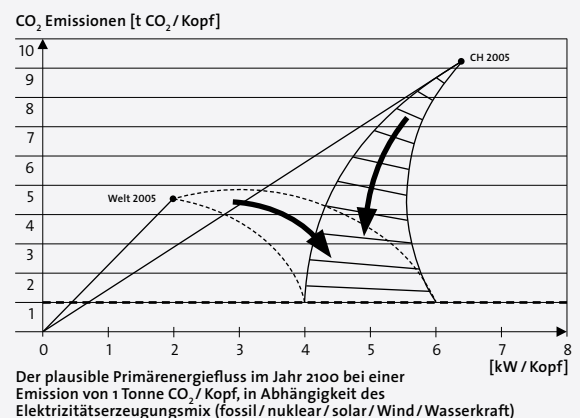
Abbildung 13: Die Emissionsgrenze für die Treibhausgase von 1 Tonne CO 2 /Kopf lässt sich gegen Ende des 21. Jahrhunderts in der Schweiz und weltweit realisieren. Dazu gilt es, die realistischen Effizienzpotenziale auszuschöpfen und alle Energiesektoren weitgehend zu entkarbonisieren.
